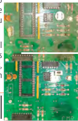
ANTES Y DESPUÉS. LIMPIEZA DE PLACA DE CIRCUITO IMPRESO
